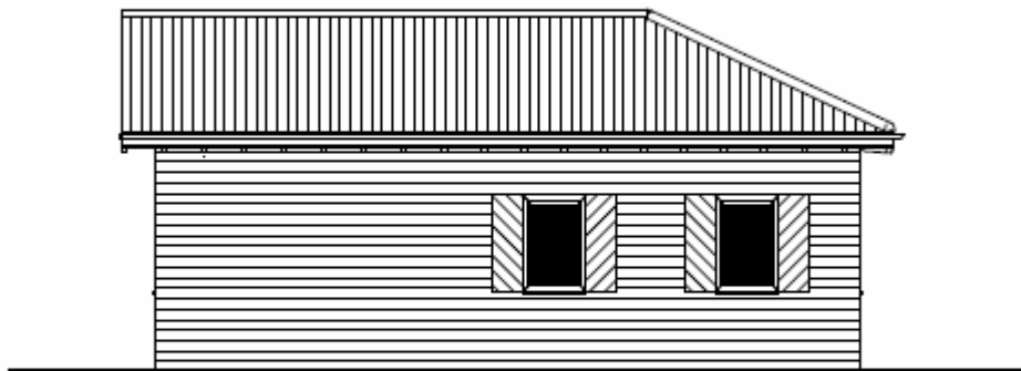
Ansicht Süd
