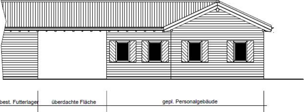
Ansicht West
