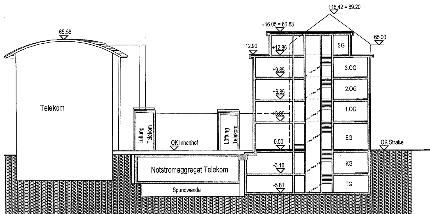
SCHNITT HOTEL
