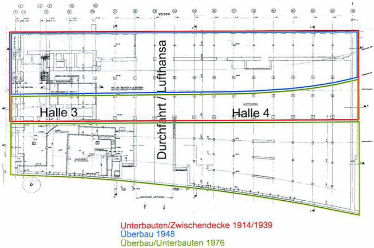
Abbildung 1: Grundriss der rechtsrheinischen Rampe
