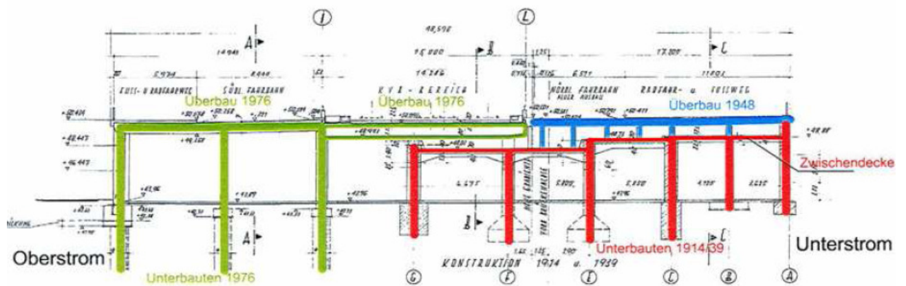
Abbildung 2: Querschnitt der rechtsrheinischen Rampe
