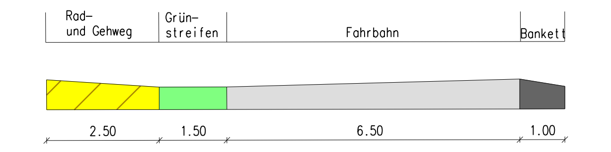
Straßenquerschnitt
