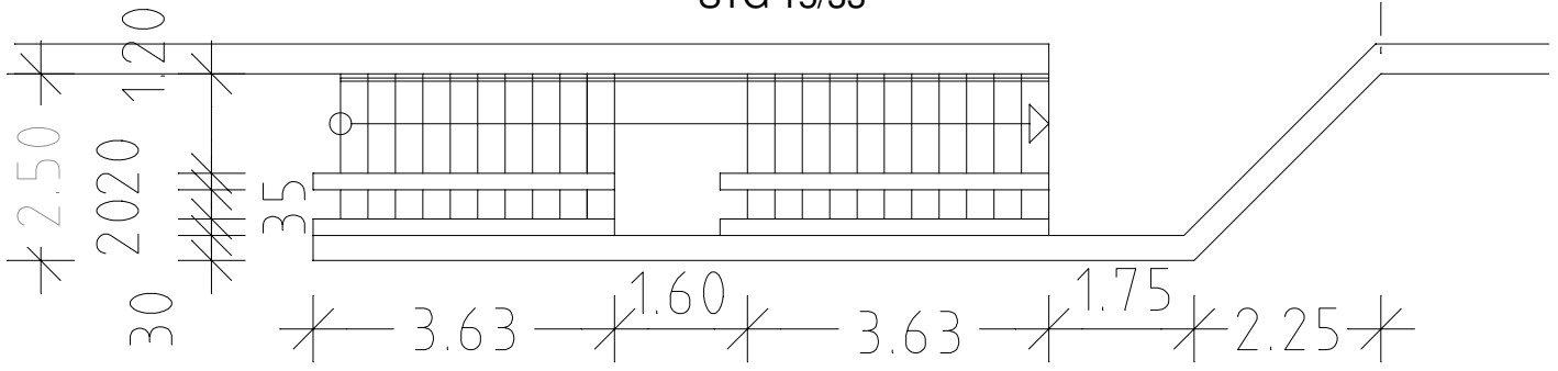
Treppe mit Fahrrad-und Kinderwagenschiene
