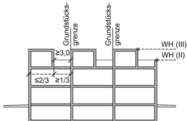
Systemschnitt WA1 und 11
