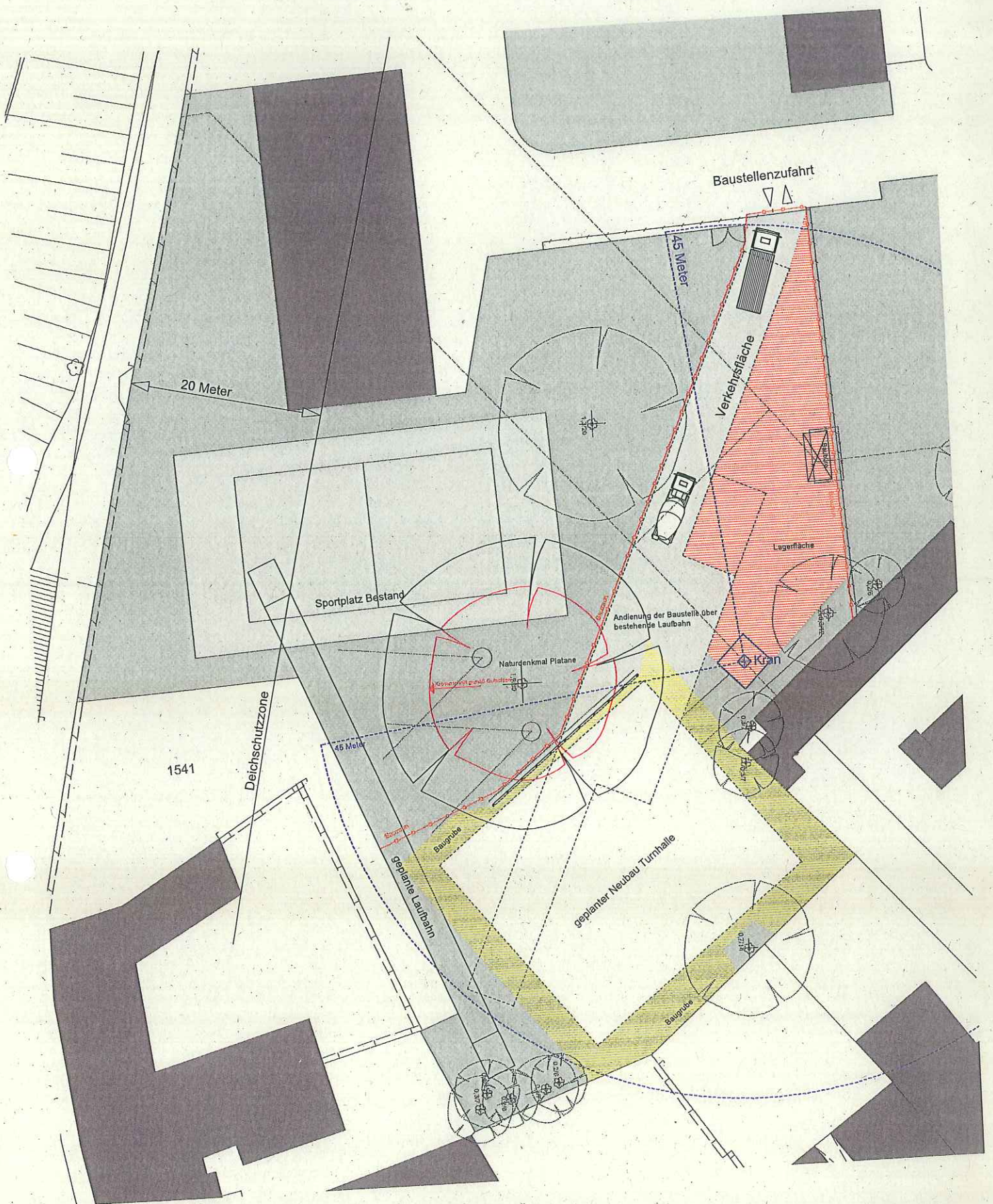
Baustelleneinrichtung M 1:500
