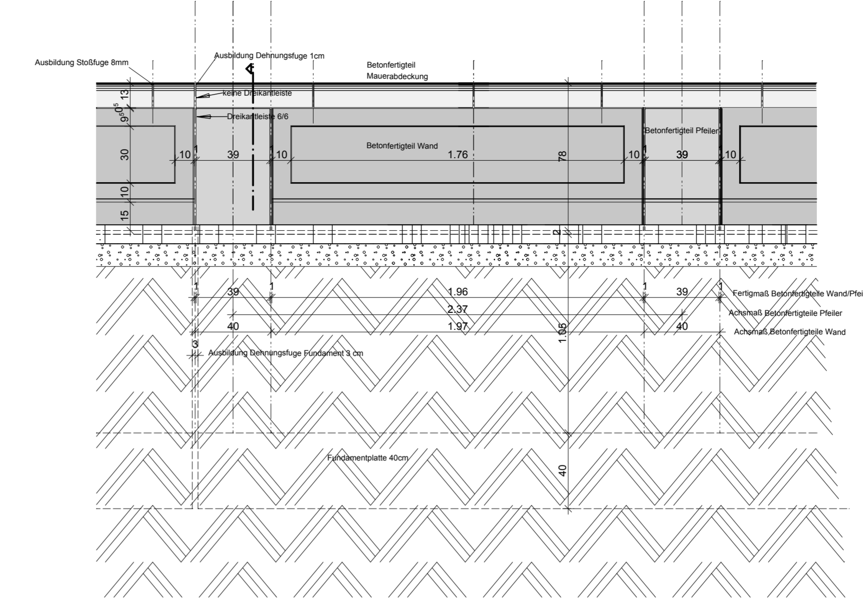
Regeldetail Betonfertigteile ANSICHT (Rechte Mauerseite)
