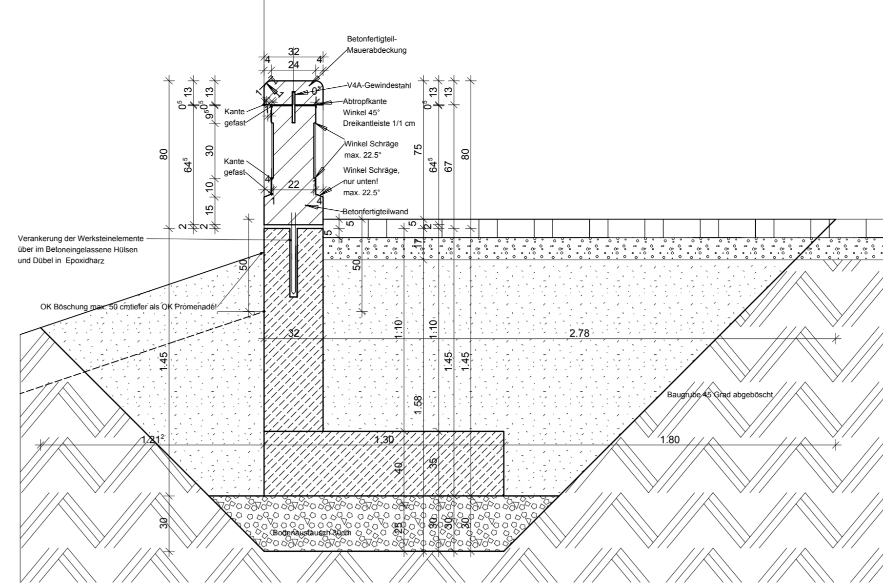
Regeldetail Betonfertigteile SCHNITT
