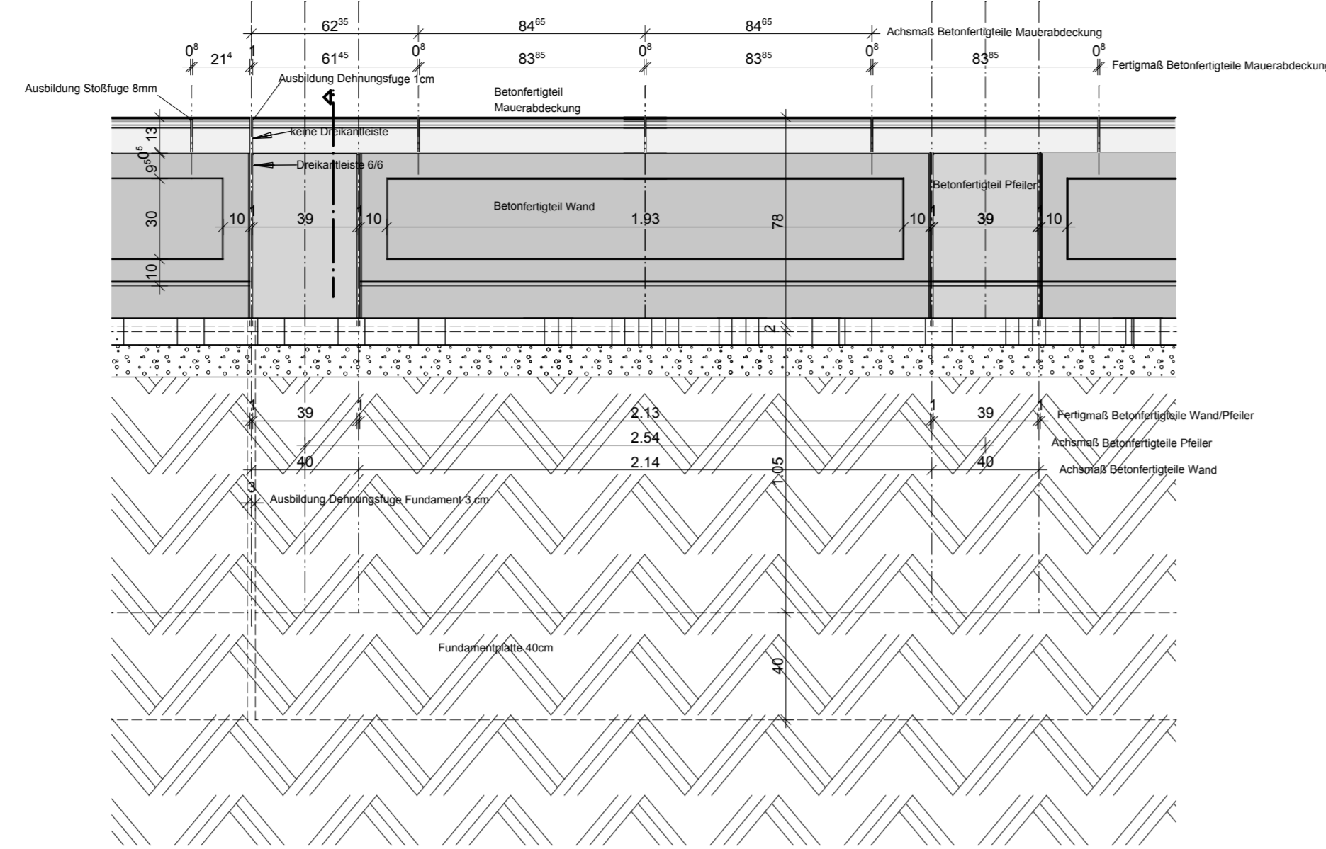
Regeldetail Betonfertigteile ANSICHT (Linke Mauerseite)
