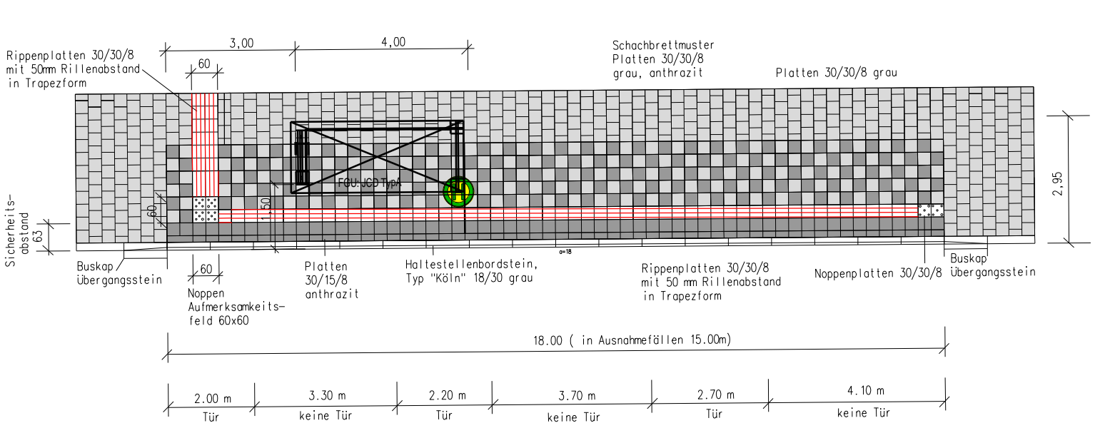
Detailzeichnung Buskap
