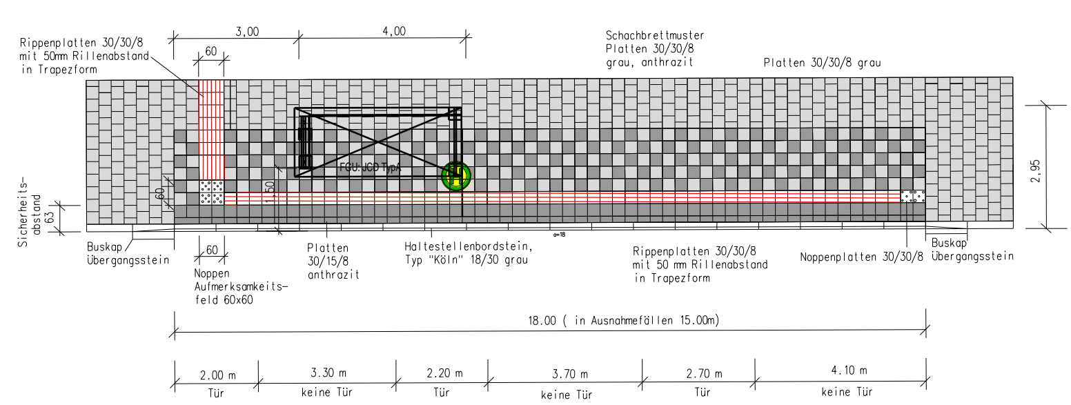
Detailzeichnung Buskap
