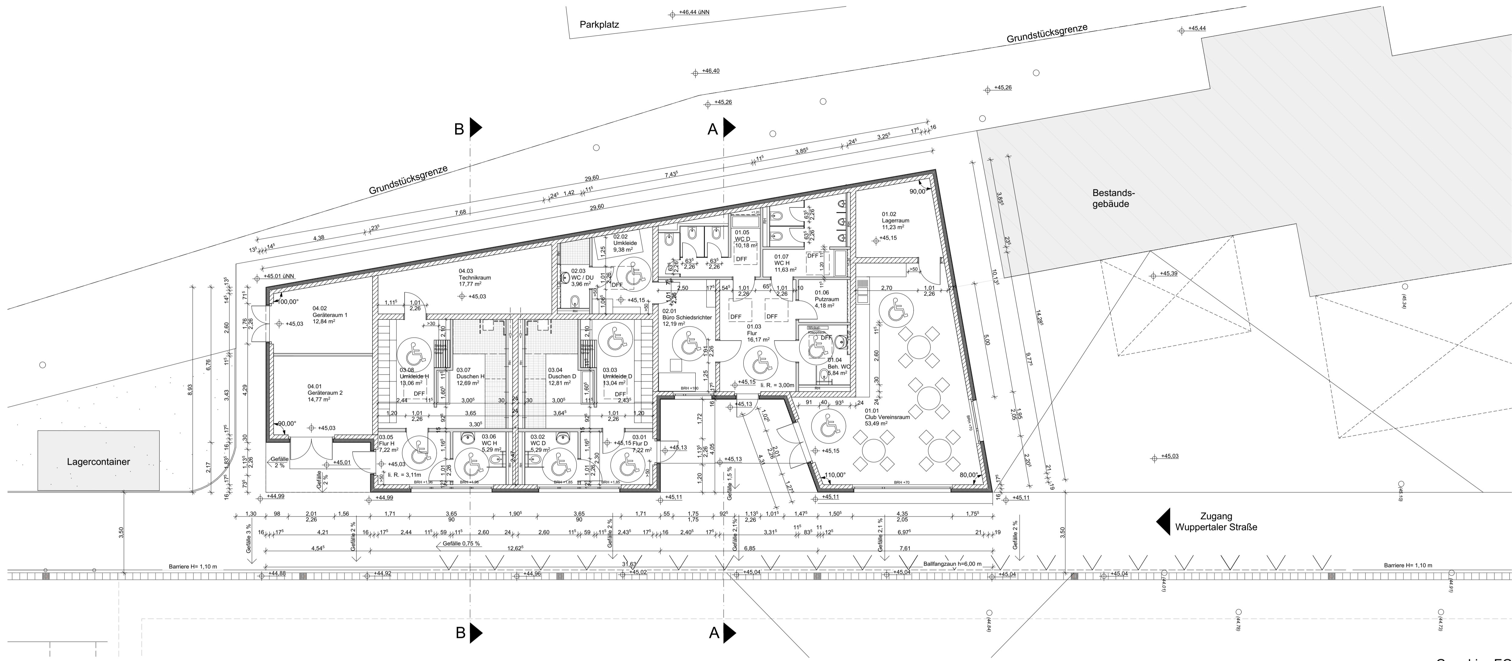
Grundriss EG
