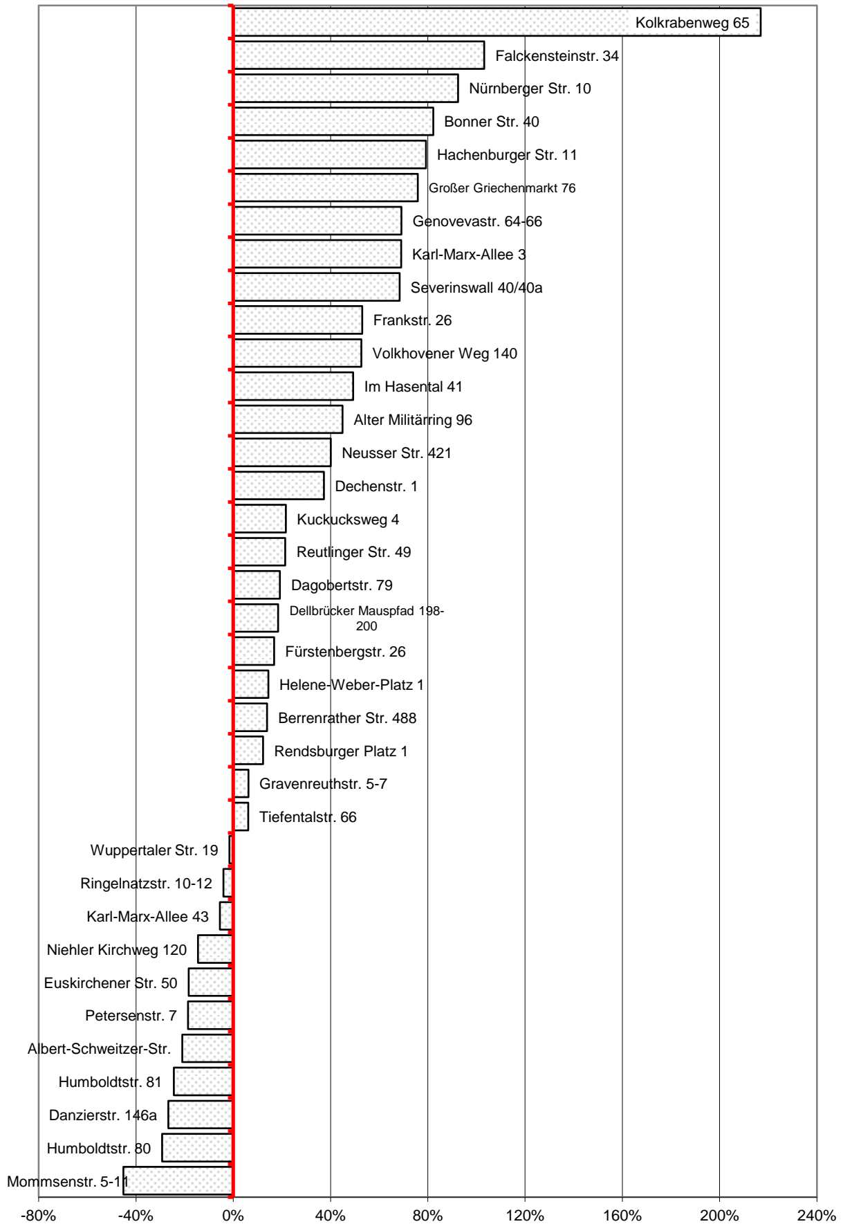
Abbildung A2.9: Haupt- und Realschulen, Heizung
