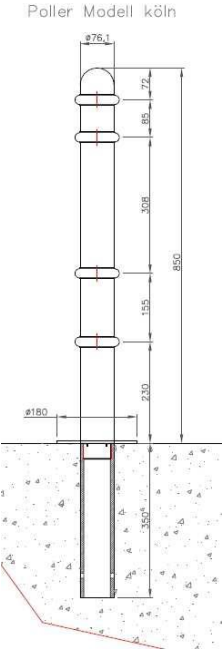
Abbildung 1: Köln Poller mit Robinson Element
