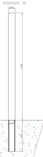
Abbildung 2: kurzer VZ-Pfosten mit Robinson-Element
