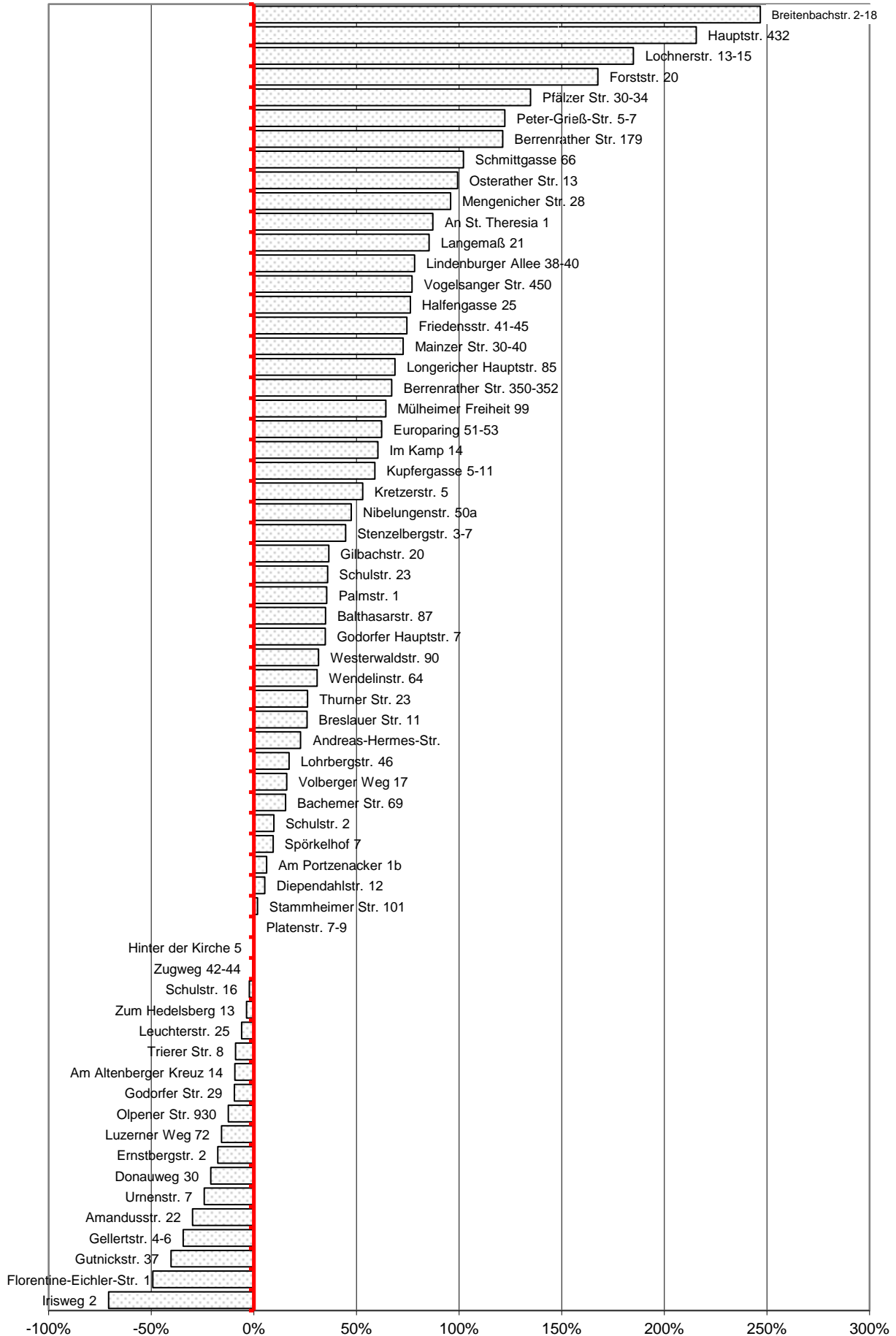
Abbildung A2.5: Grundschulen <math><3.500\text{ m}^2</math>, Heizung
