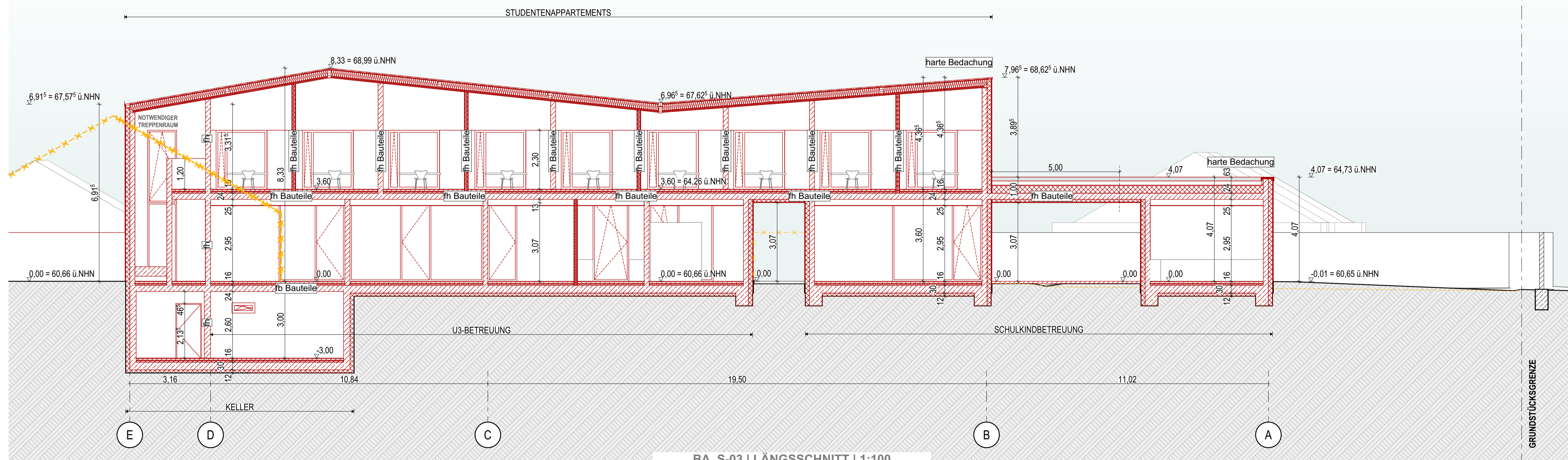
BA_S-03 | LÄNGSSCHNITT | 1:100
