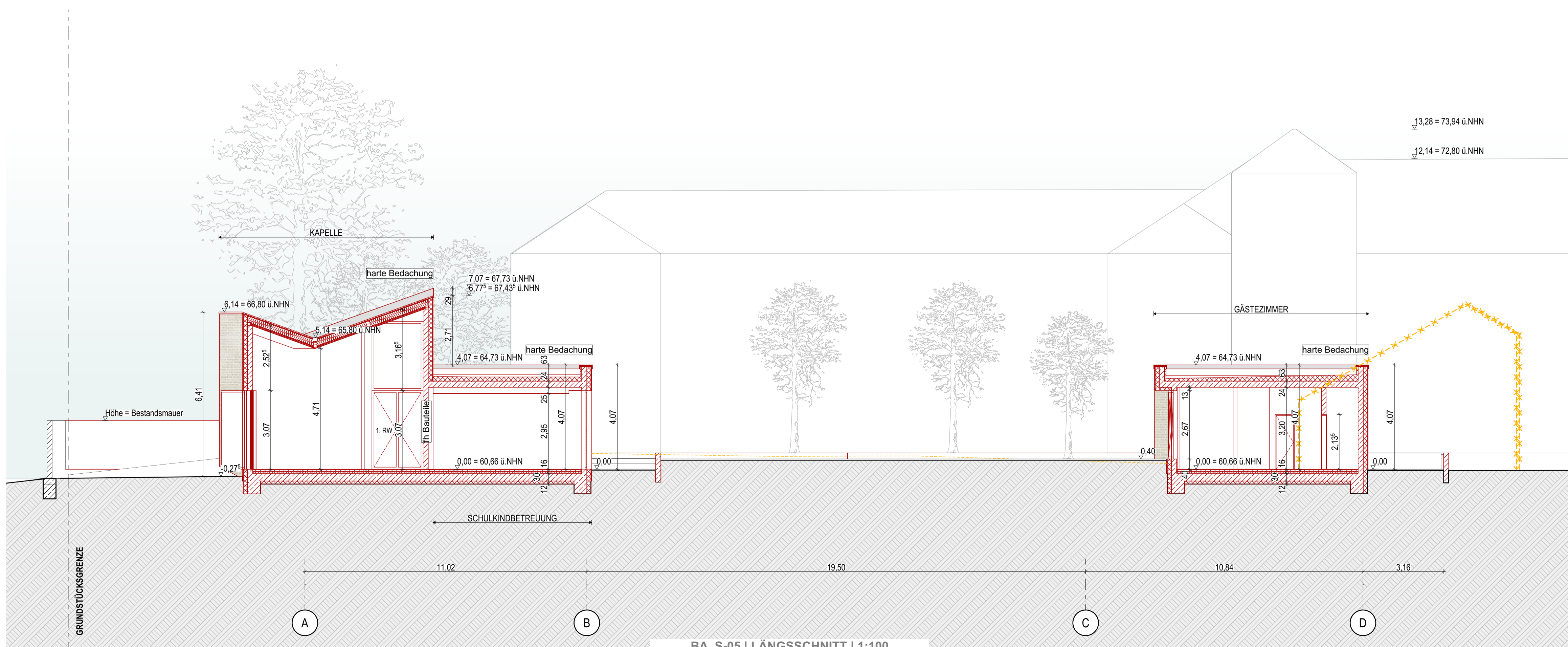
BA_S-05 | LÄNGSSCHNITT | 1:100
