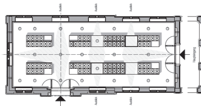
Entwurf 03, Grundriss, Melatenfriedhof
