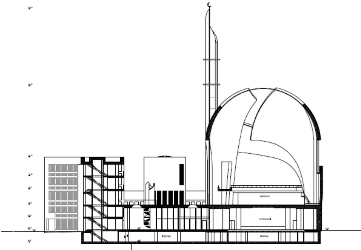
Schnitt Fuchsstraße / Innere Kanalstraße (Moschee)
