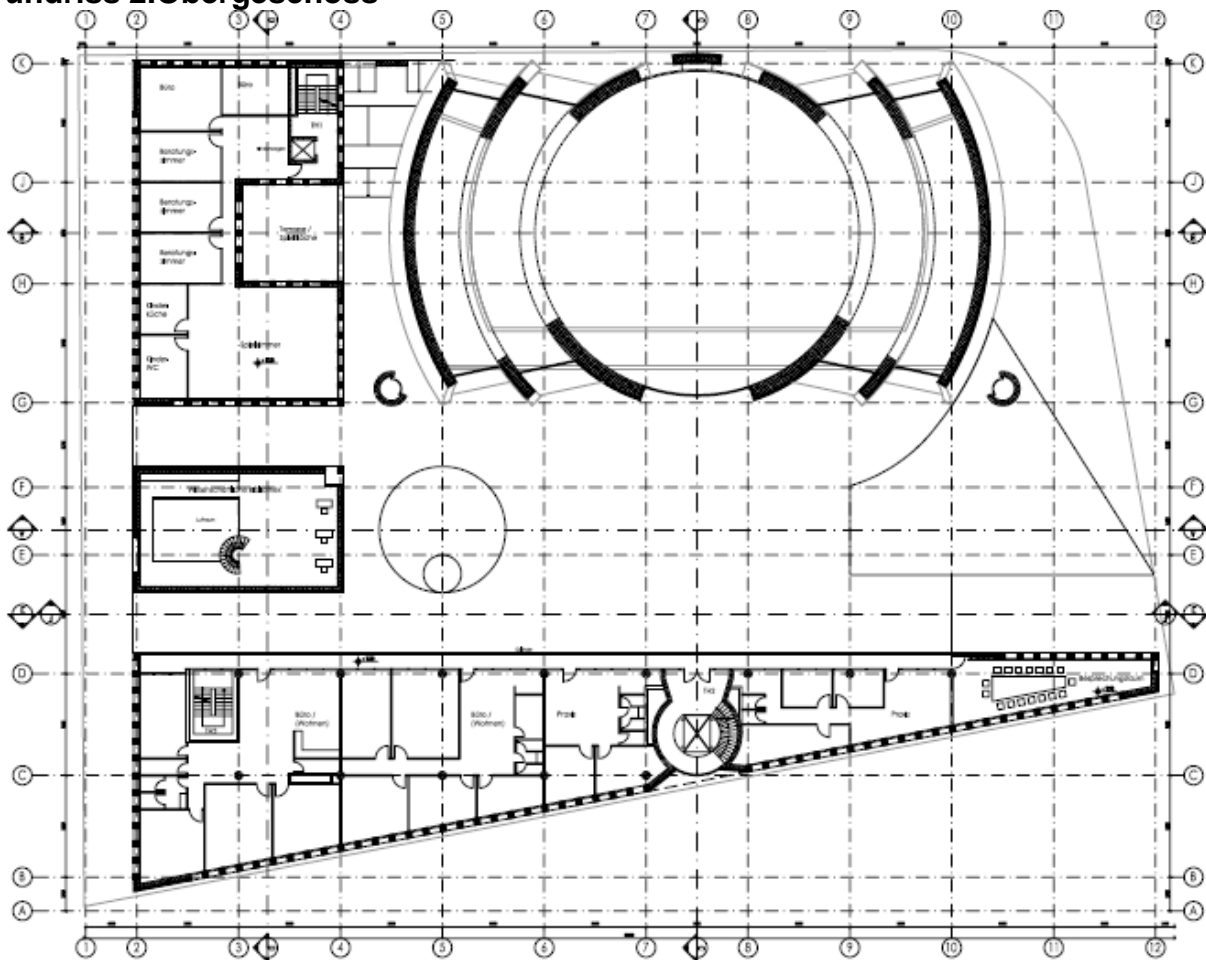
Grundriss 3. Obergeschoss
