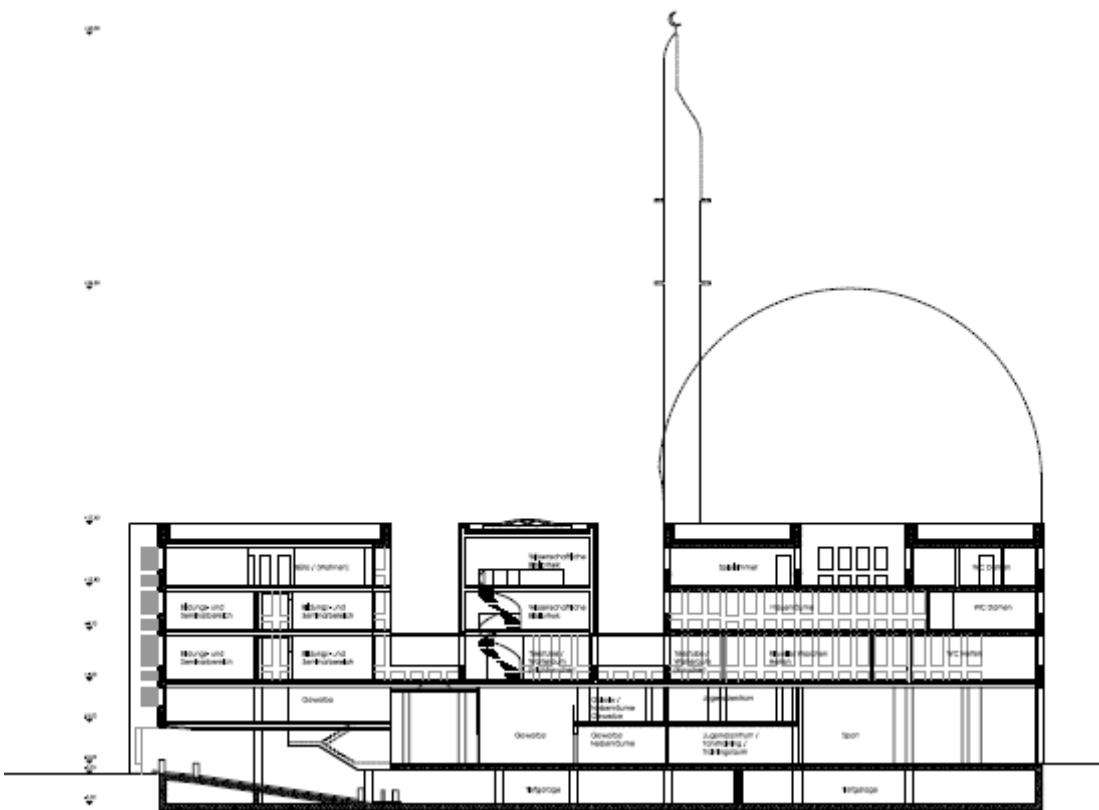
Schnitt Fuchsstraße / Innere Kanalstraße (Verwaltungstrakt)
