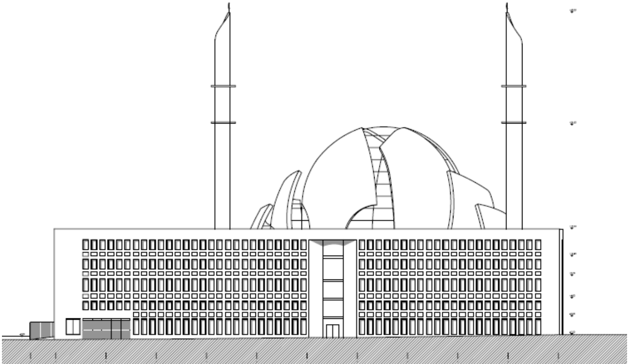
Ansicht Fuchsstraße
