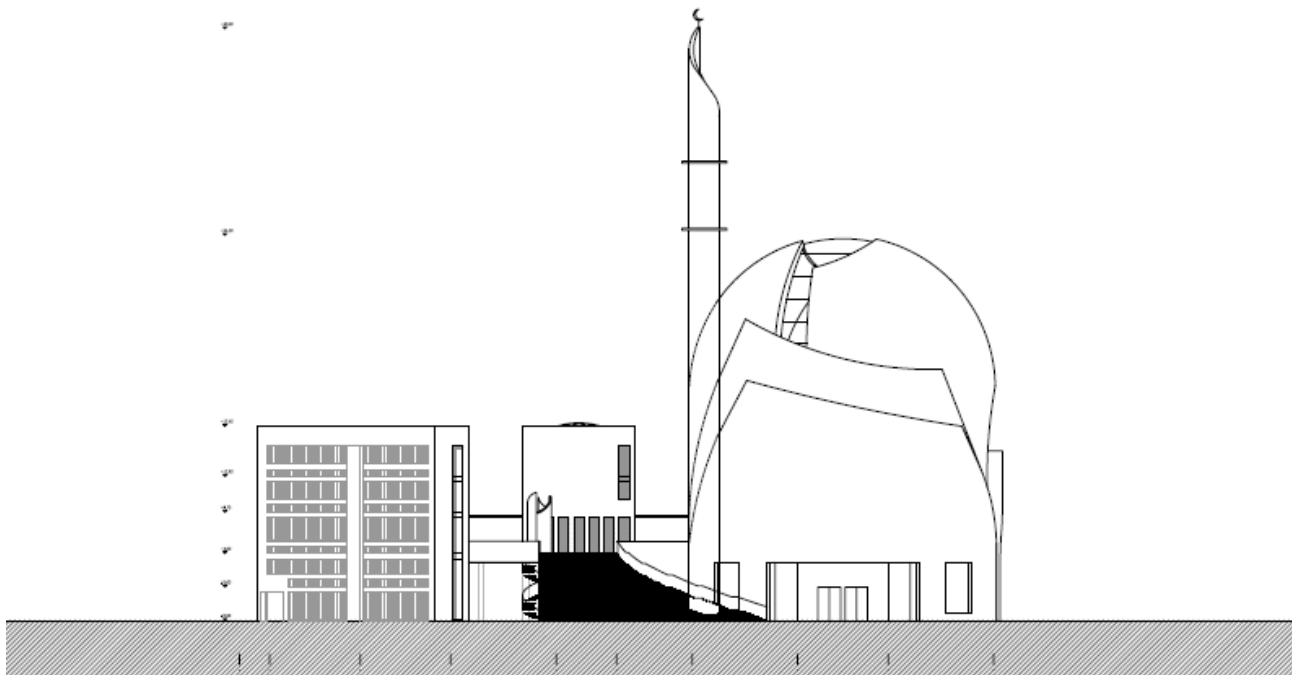
Ansicht Venloer Straße
