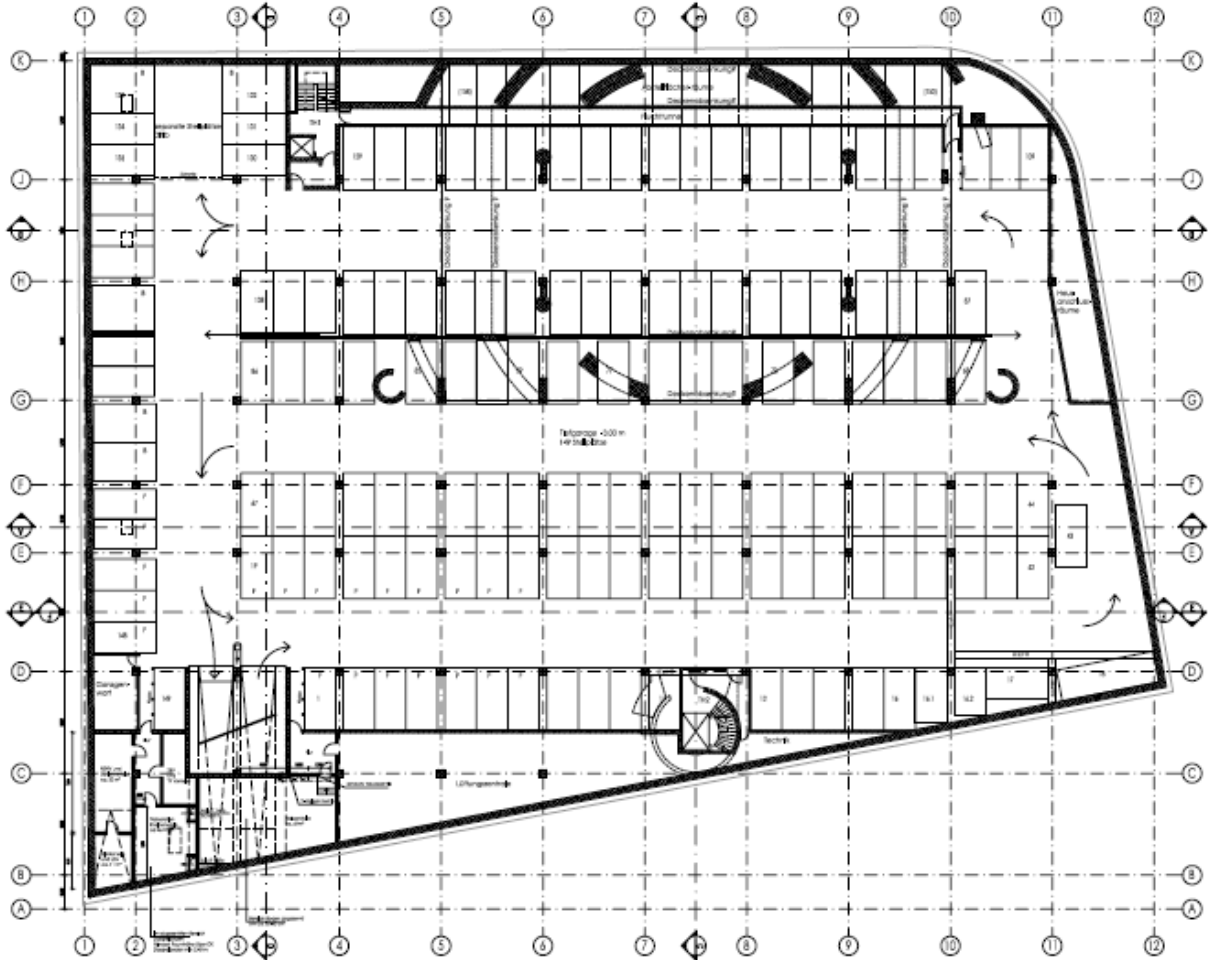
Grundriss Tiefgarage
