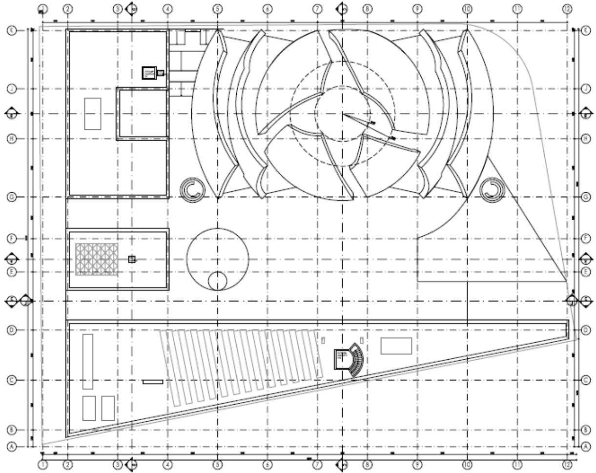
Dachaufsicht
