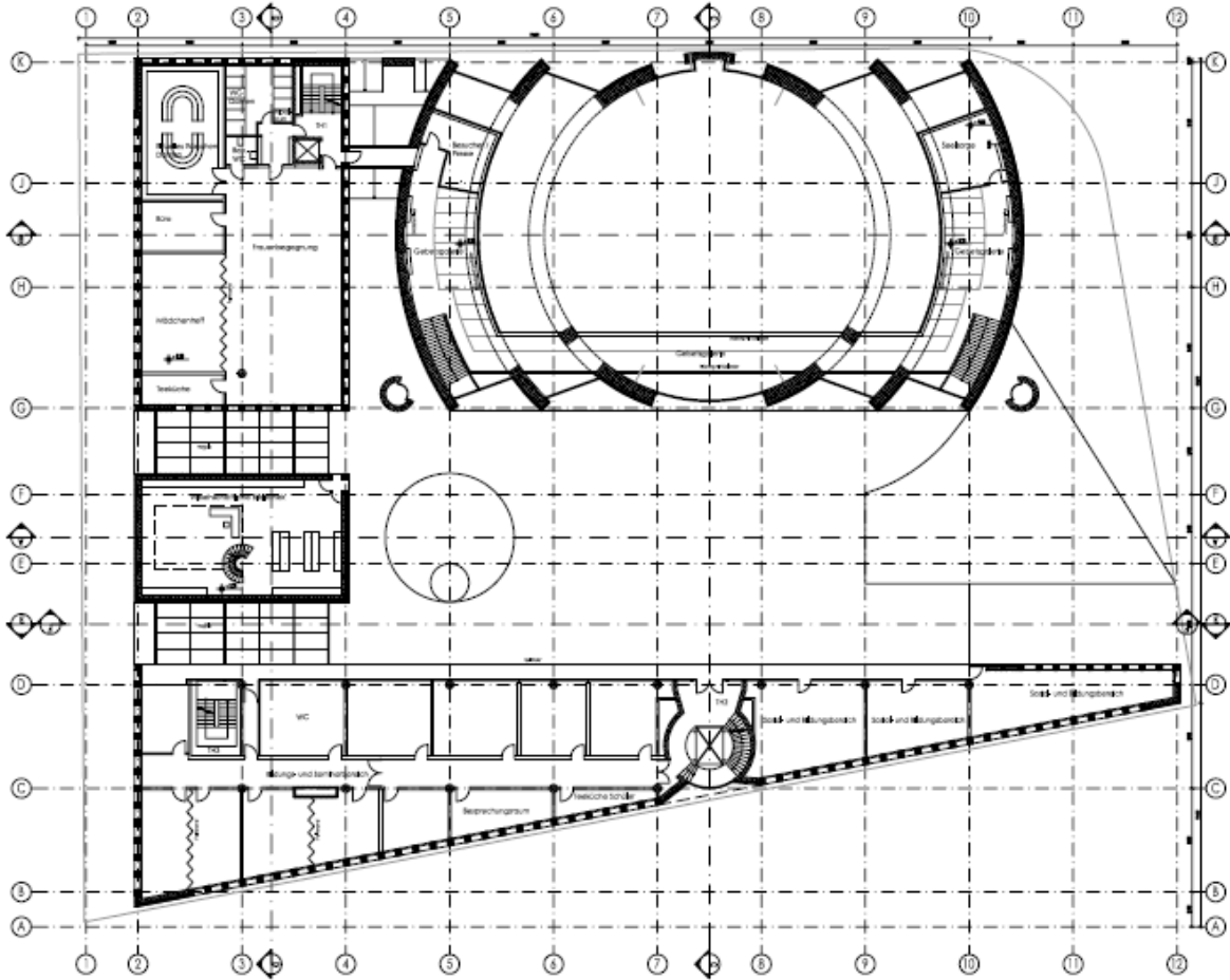
Grundriss 2. Obergeschoss
