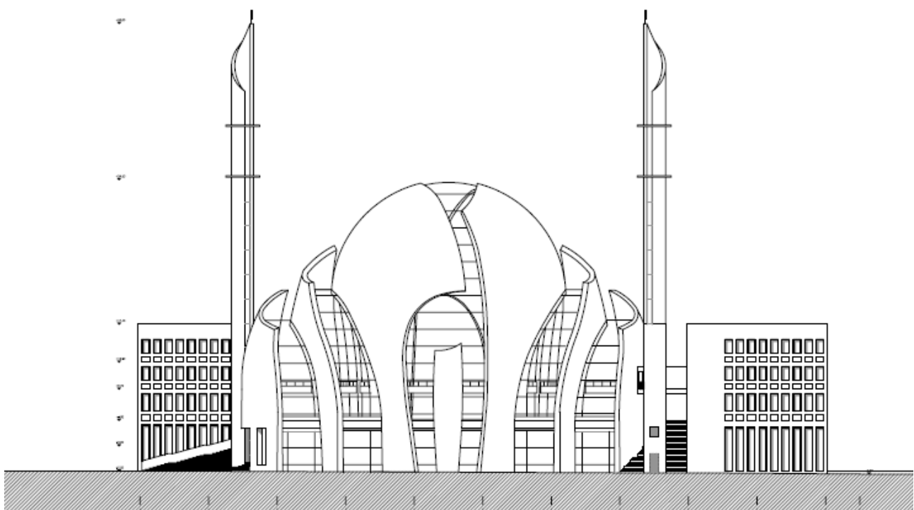
Ansicht Innere Kanalstraße
