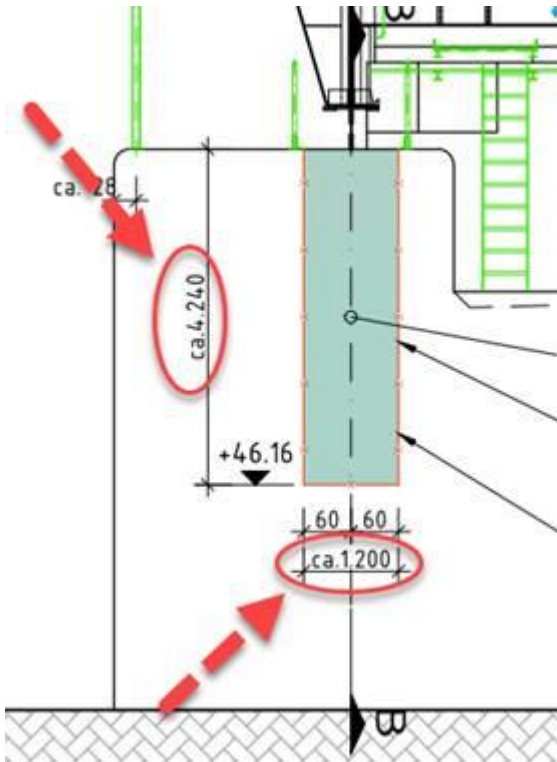
Bild 1: Ausschnitt aus dem Ausführungsplan Ankerpfeiler
